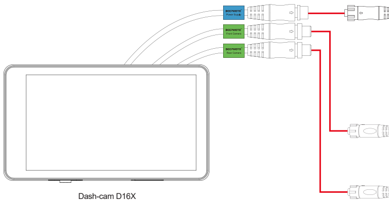
Dash-cam D16X
